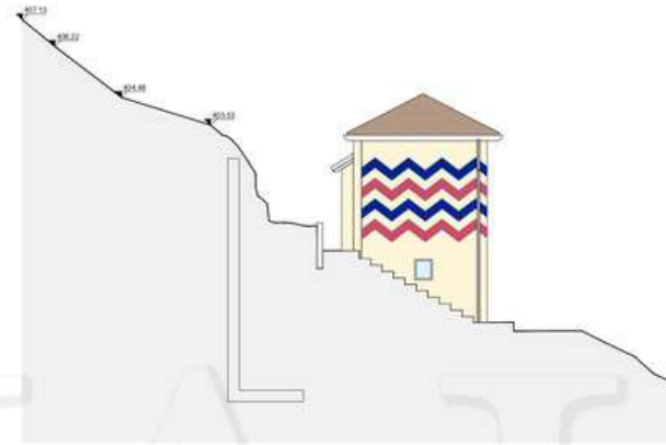
PROSPETTO OVEST
